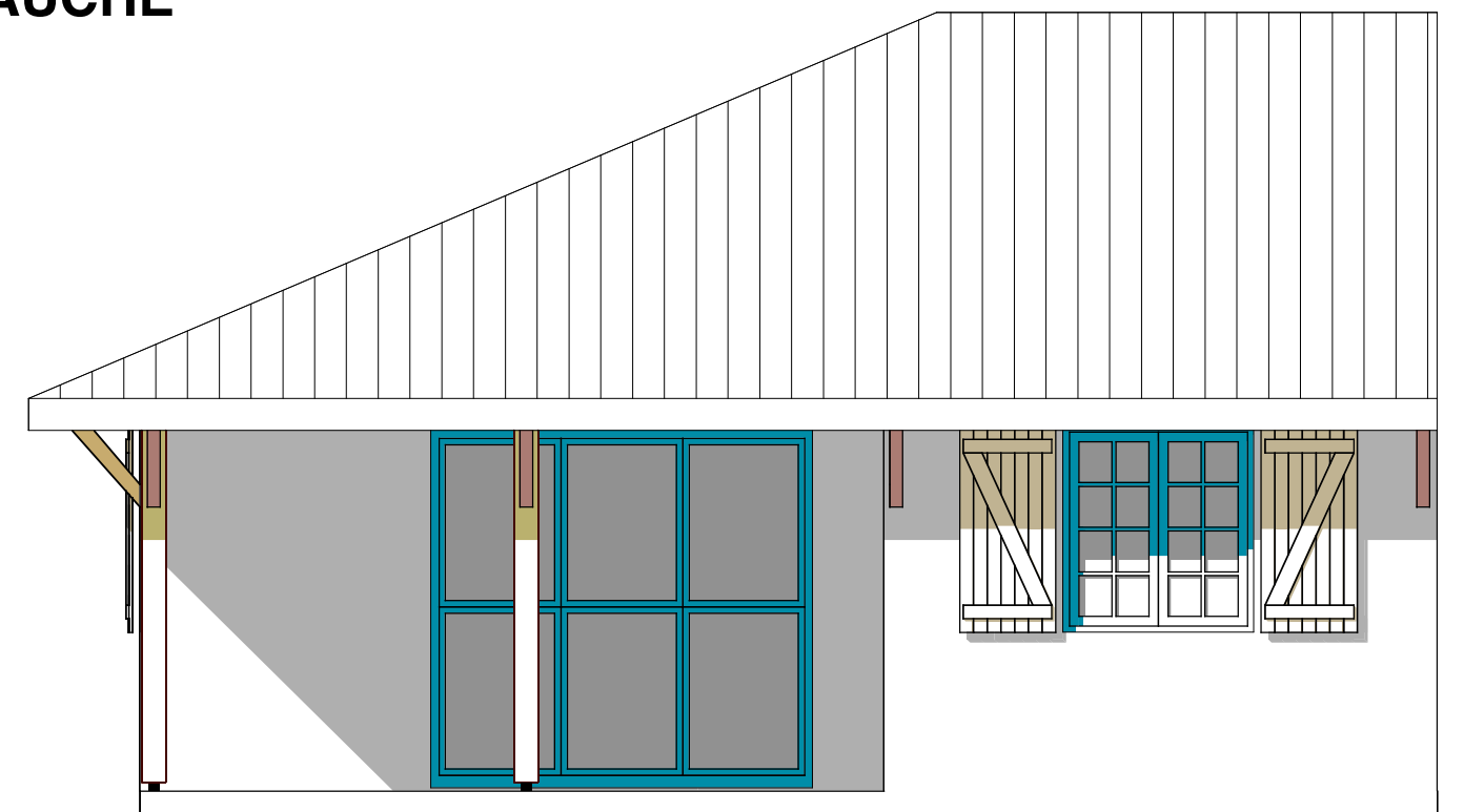
PIGNON GAUCHE
